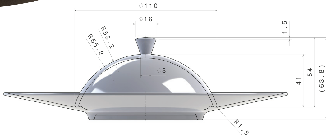
Coupe A-A Echelle : 1:1
