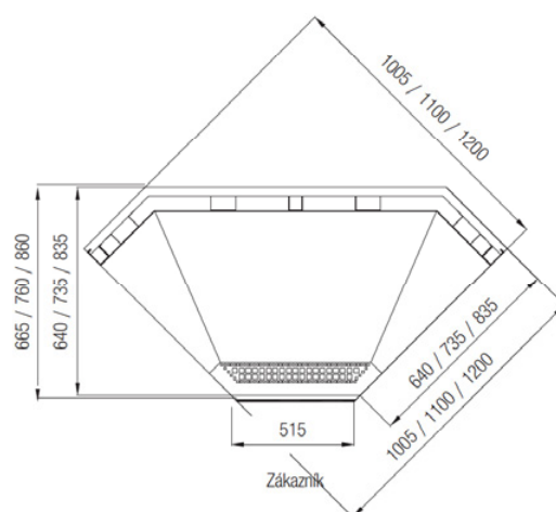
Bokorys rohu
