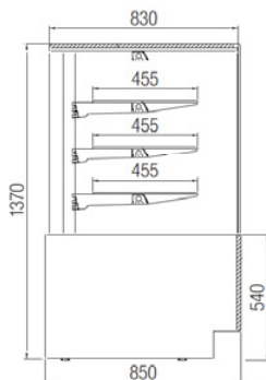
Bokorys Raffaello
