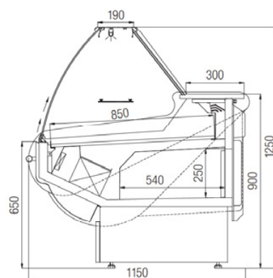
Verze W – ventilovaná
