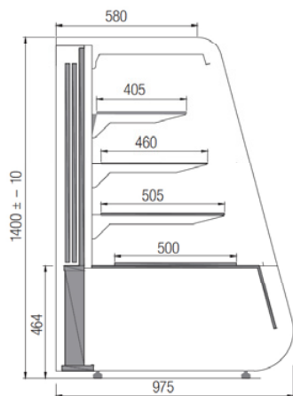
Bokorys Dolce
