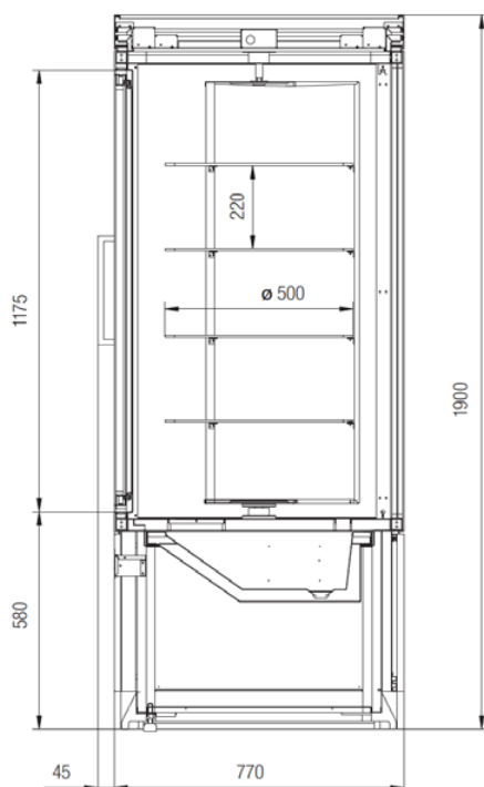
Bokorys Ardea
