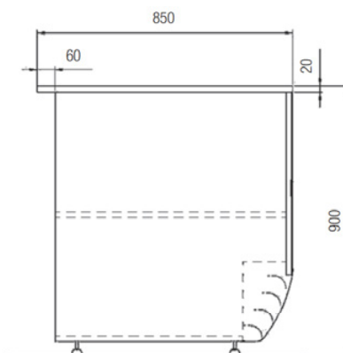
Neutrální pult
