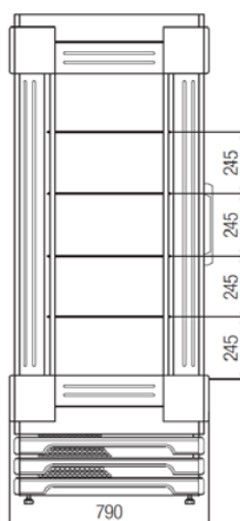
Boční pohled
