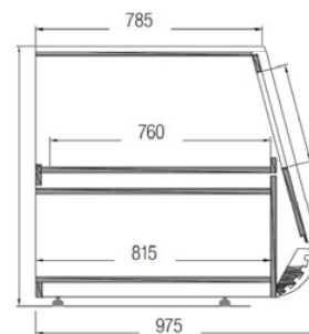
Neutrální pult
