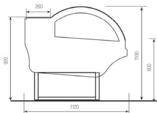
Neutrální pult
