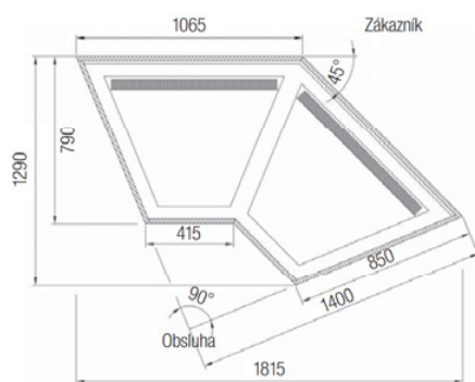
Roh 90° otevřený ventilovaný
