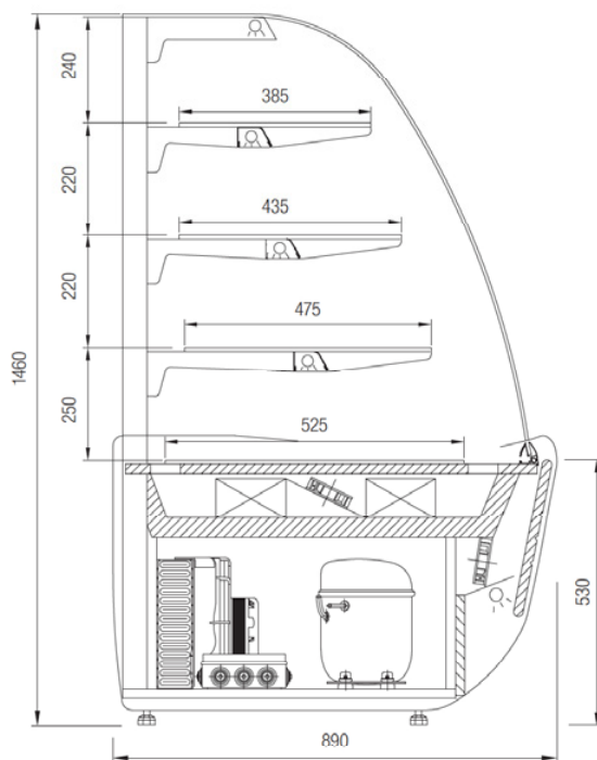
Bokorys Bellissima CH
