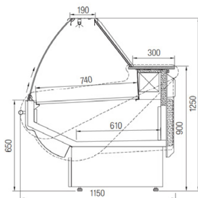
Verze G – statická
