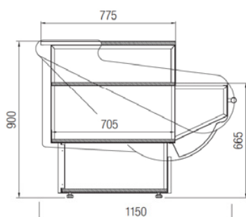
Neutrální pult
