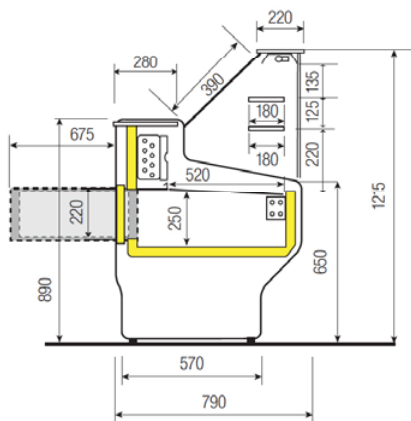
Hill HD – rovné kolmé sklo
