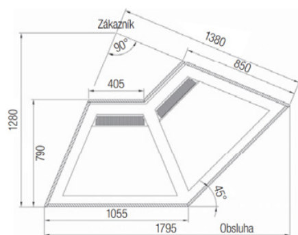
Roh 90° uzavřený ventilovaný
