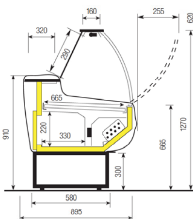
Ventilovaná verze BC s výklopným sklem CY
