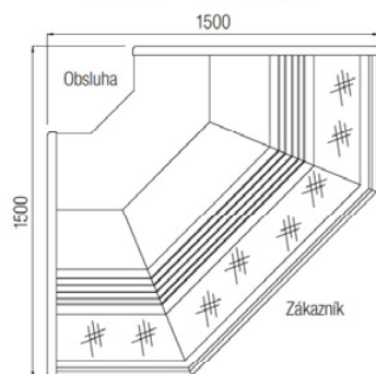
Roh 90° otevřený ventilovaný
