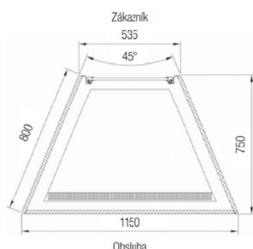
Roh 45° uzavřený ventilovaný
