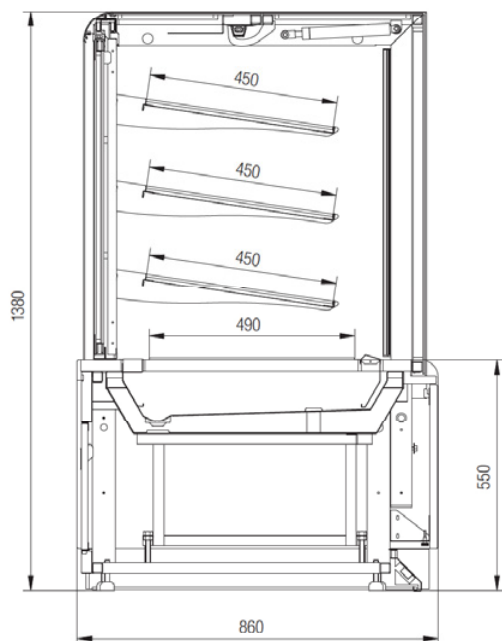
Bokorys Limicola
