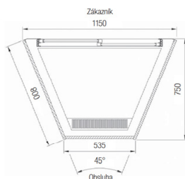
Roh 45° otevřený ventilovaný
