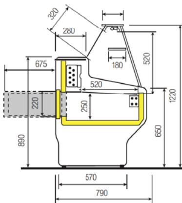
Hill HL – rovné šikmé sklo
