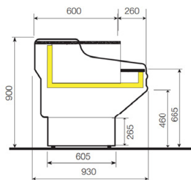
Neutrální pult
