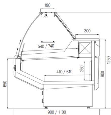
Verze G – statická
