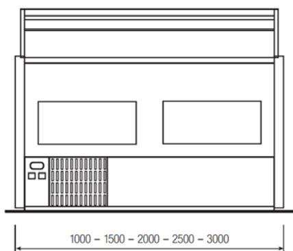
Zadní pohled
