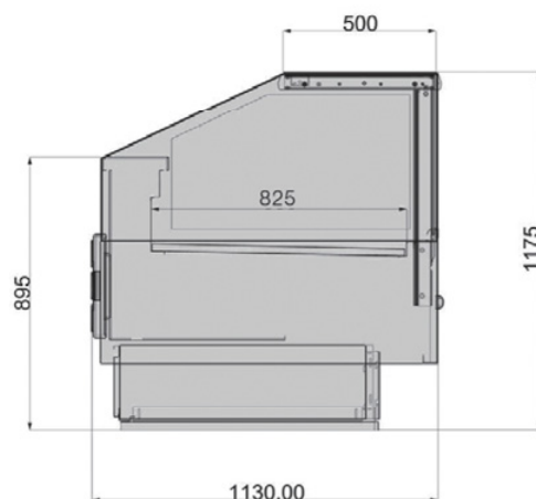
Bokorys Musca
