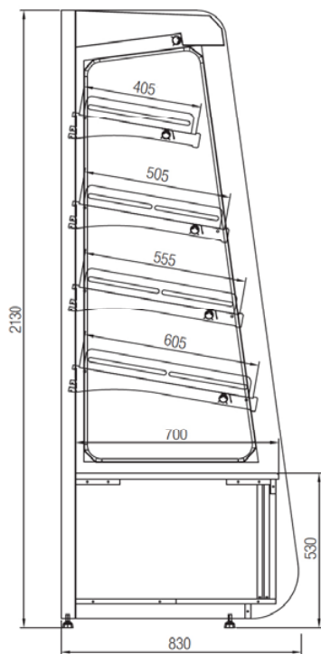
Bokorys R Dolce A
