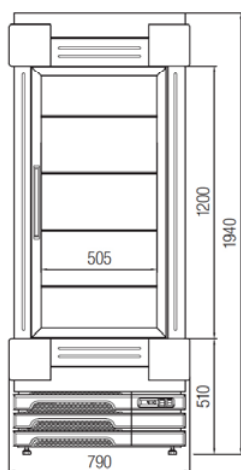
Čelní pohled
