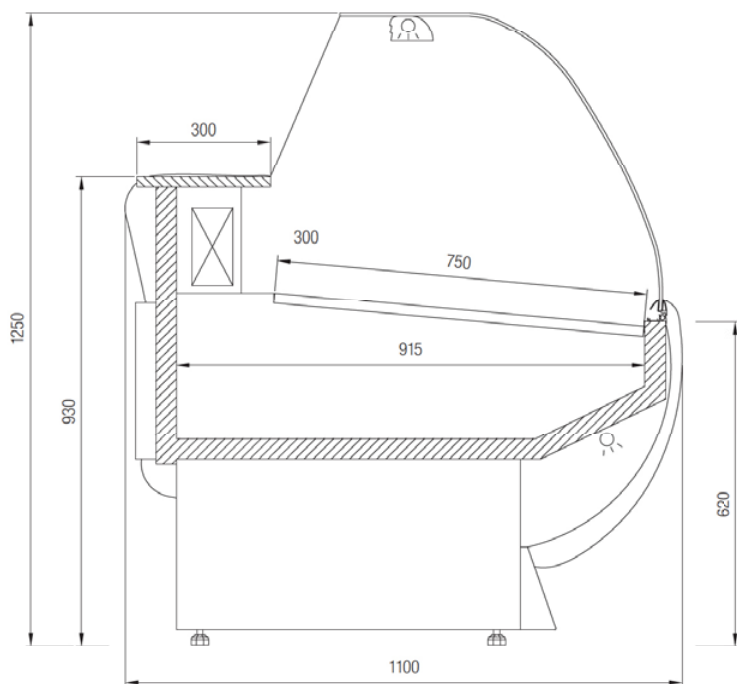
Bokorys Europa
