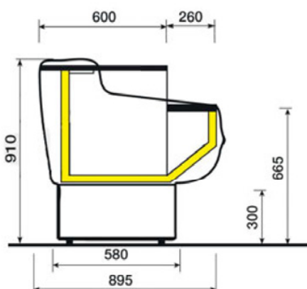
Neutrální pult
