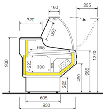
Ventilovaná verze BC s oblým sklem JY
