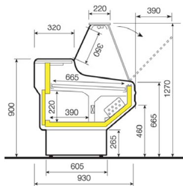
Ventilovaná verze BC s šikmým sklem JD
