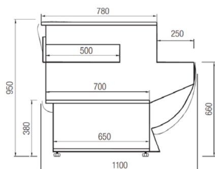
Neutrální pult
