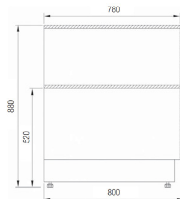
Neutrální pult
