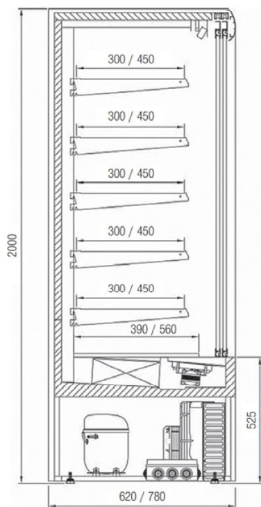
Verze s dveřmi
