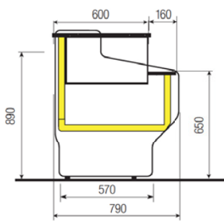
Neutrální pult
